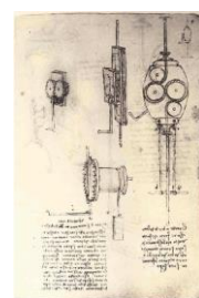
Léonard de Vinci Etude de poulis Codex de Madrid I 1490-99 Dessin
